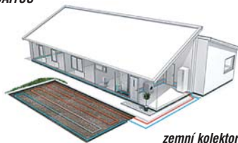
zemní kolektor
